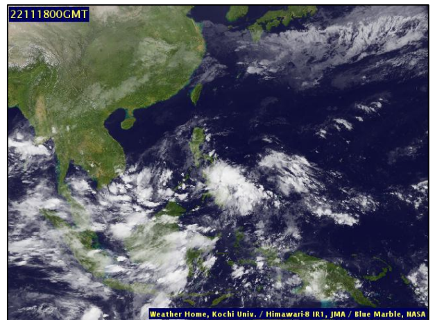
ภาพถ่ายดาวเทียม วันที่ ๑๘ พ.ย. ๒๕๖๕ เวลา ๐๗.๐๐ น.
