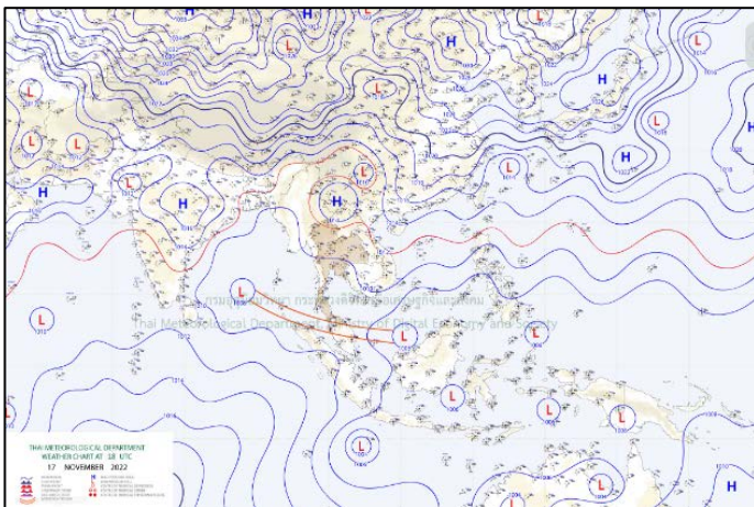
แผนที่อากาศ วันที่ ๑๘ พ.ย. ๒๕๖๕ เวลา ๐๑.๐๐ น.
