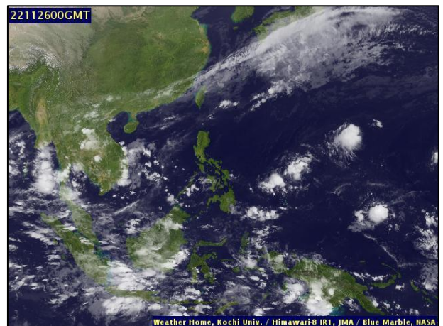
ภาพถ่ายดาวเทียม วันที่ ๒๖ พ.ย. ๒๕๖๕ เวลา ๐๗.๐๐ น.
