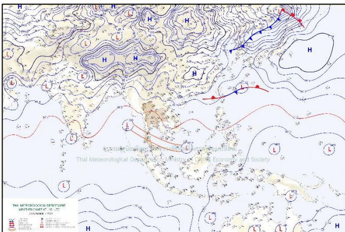
แผนที่อากาศ วันที่ ๒๖ พ.ย. ๒๕๖๕ เวลา ๐๑.๐๐ น.
