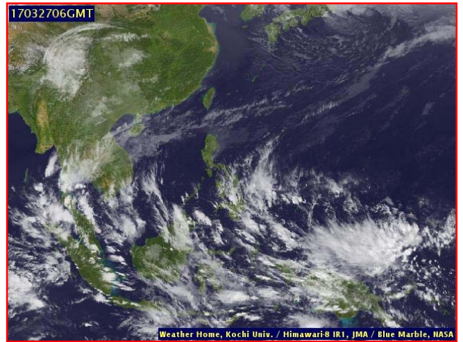
ภาพถ่ายจากดาวเทียม วันที่ ๒๗ มี.ค. ๒๕๖๐ เวลา ๑๓.๐๐ น.
