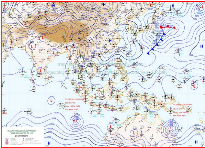
แผนที่อากาศ วันที่ ๒๗ มี.ค. ๒๕๖๐ เวลา ๐๗.๐๐ น.
