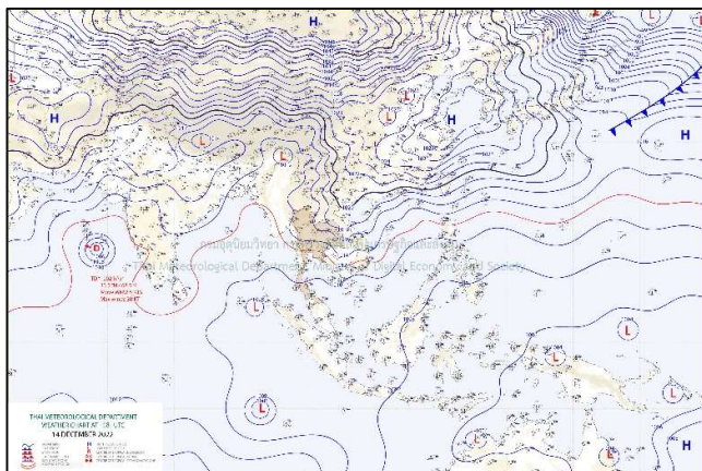
แผนที่อากาศ วันที่ ๑๕ ธ.ค. ๒๕๖๕ เวลา ๐๑.๐๐ น.
