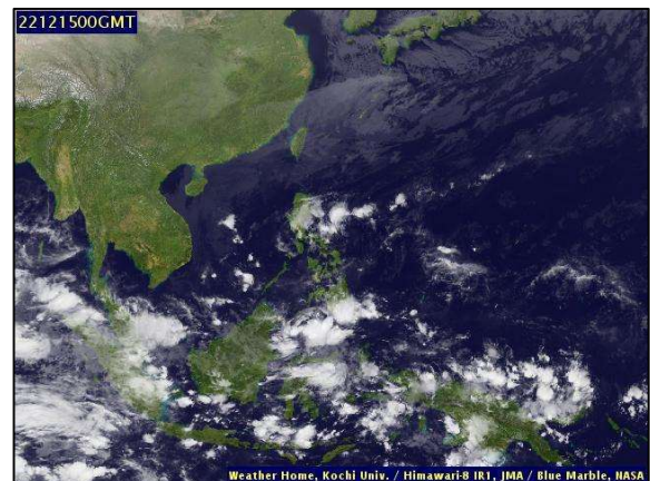
ภาพถ่ายดาวเทียม วันที่ ๑๕ ธ.ค. ๒๕๖๕ เวลา ๐๗.๐๐ น.
