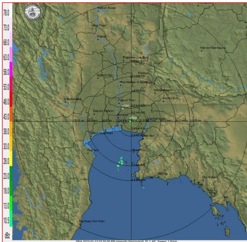
ภาพเรดาร์ตรวจอากาศ “สถานีสุวรรณภูมิ” ณ วันที่ 13 มกราคม 2566 เวลา 10.30 น. (ที่มา : กรมอุตุนิยมวิทยา)
