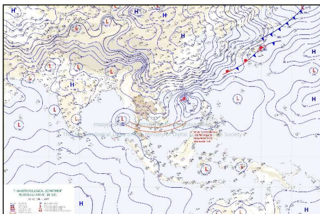
แผนที่อากาศ วันที่ ๑๙ ม.ค. ๒๕๖๖ เวลา ๐๗.๐๐ น.
