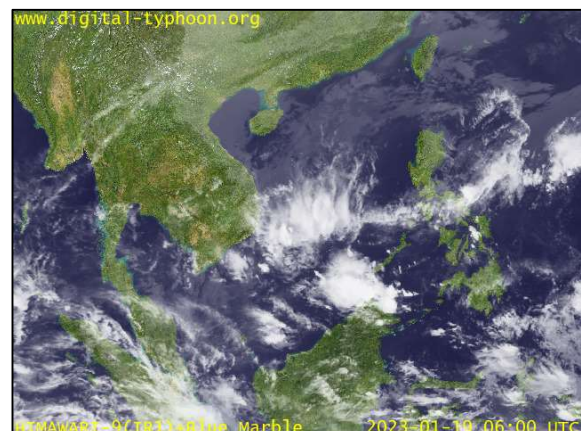
ภาพถ่ายดาวเทียม วันที่ ๑๙ ม.ค. ๒๕๖๖ เวลา ๑๓.๐๐ น.
