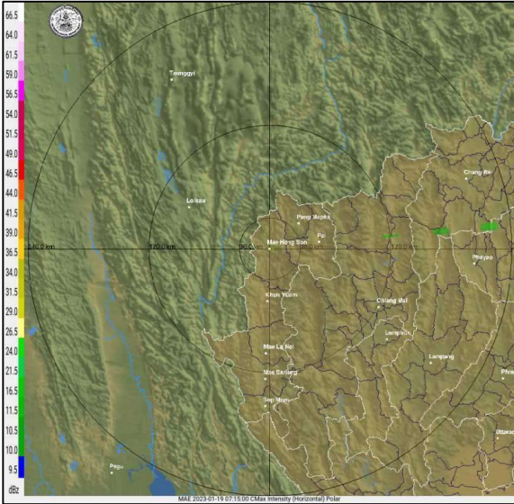
สถานีแม่ฮ่องสอน เวลา ๑๔.๑๕ น.
