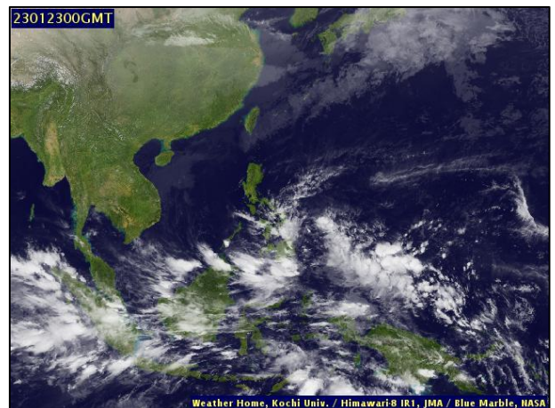
ภาพถ่ายดาวเทียม วันที่ ๒๓ ม.ค. ๒๕๖๖ เวลา ๐๗.๐๐ น.
