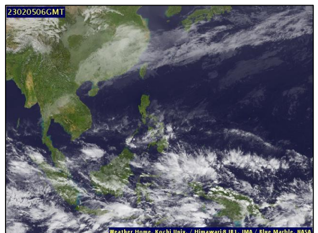
ภาพถ่ายดาวเทียม วันที่ ๕ ก.พ. ๒๕๖๖ เวลา ๑๓.๐๐ น.
