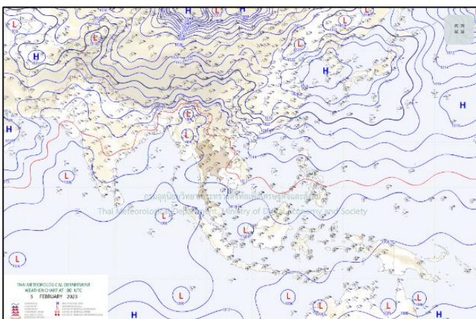
แผนที่อากาศ วันที่ ๕ ก.พ. ๒๕๖๖ เวลา ๐๗.๐๐ น.
