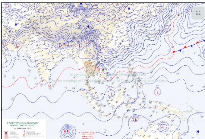
แผนที่อากาศ วันที่ ๑๕ ก.พ. ๒๕๖๖ เวลา ๐๑.๐๐ น.
