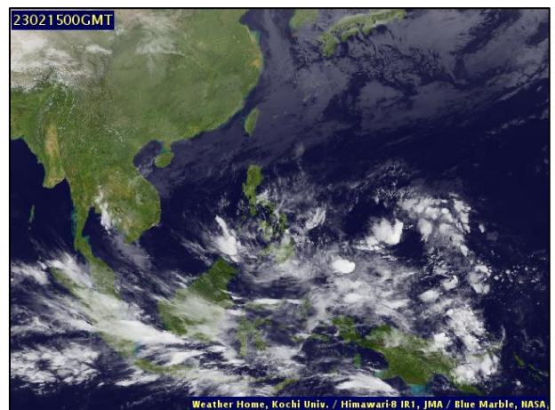
ภาพถ่ายดาวเทียม วันที่ ๑๕ ก.พ. ๒๕๖๖ เวลา ๐๗.๐๐ น.
