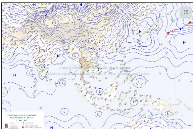
แผนที่อากาศ วันที่ ๒ พ.ค. ๒๕๖๖ เวลา ๐๑.๐๐ น.
