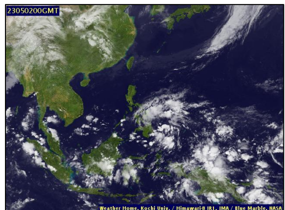
ภาพถ่ายดาวเทียม วันที่ ๒ พ.ค. ๒๕๖๖ เวลา ๐๗.๐๐ น.
