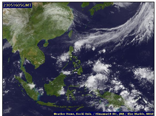
ภาพถ่ายดาวเทียม วันที่ ๑๖ พ.ค. ๒๕๖๖ เวลา ๑๒.๐๐ น.
