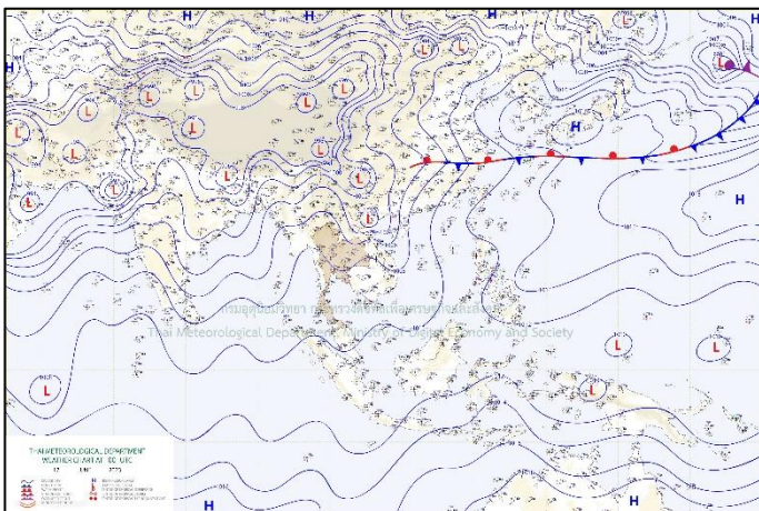
แผนที่อากาศ วันที่ ๑๗ มิ.ย. ๒๕๖๖ เวลา ๐๗.๐๐ น.
