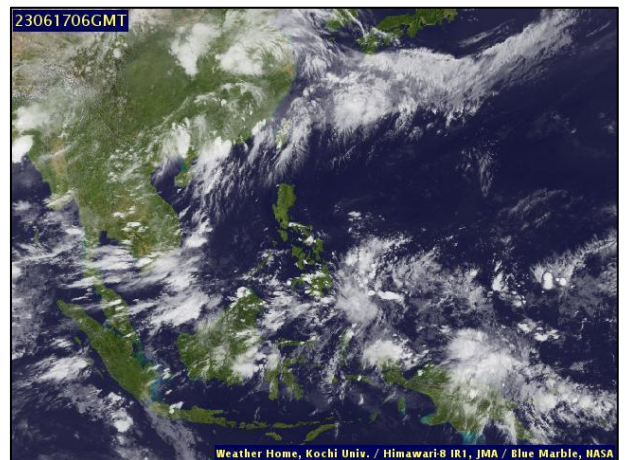
ภาพถ่ายดาวเทียม วันที่ ๑๗ มิ.ย. ๒๕๖๖ เวลา ๑๓.๐๐ น.
