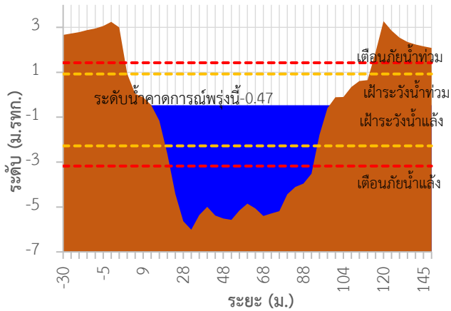
TC191802 สะพานบ้านโรงเหล็ก
