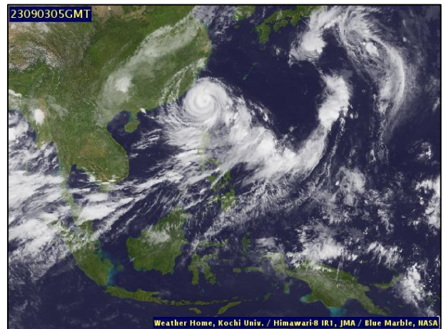
ภาพถ่ายดาวเทียม วันที่ ๓ ก.ย. ๖๖ เวลา ๑๒.๐๐ น.
