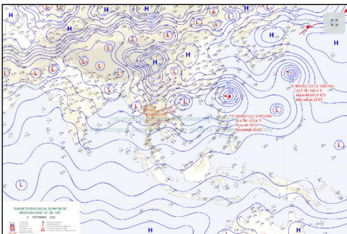
แผนที่อากาศ วันที่ ๓ ก.ย. ๒๕๖๖ เวลา ๐๗.๐๐ น.
