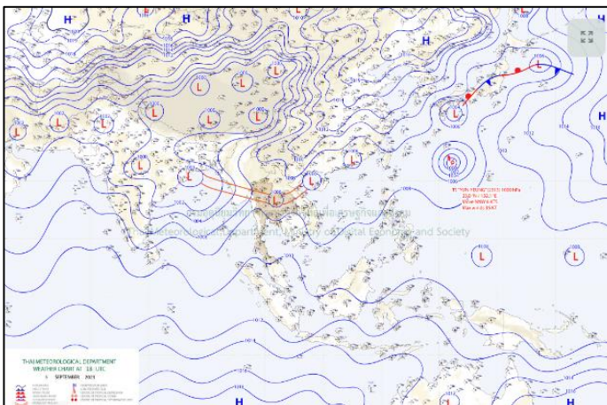
แผนที่อากาศ วันที่ ๖ ก.ย. ๒๕๖๖ เวลา ๐๑.๐๐ น.
