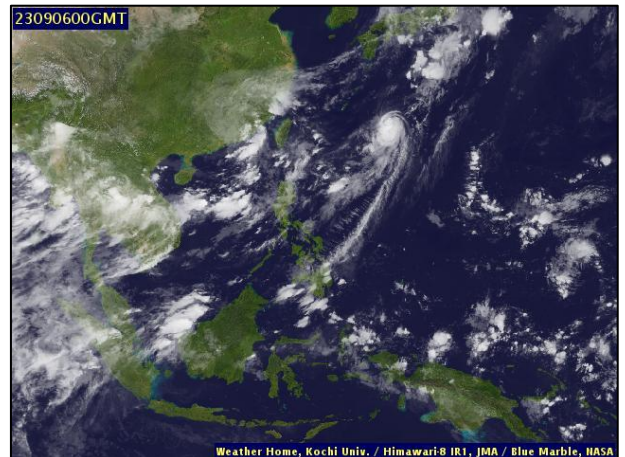
ภาพถ่ายดาวเทียม วันที่ ๖ ก.ย. ๖๖ เวลา ๐๗.๐๐ น.
