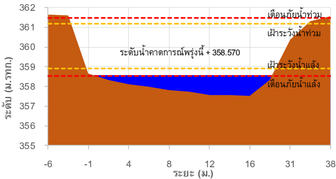
TC 020903 สะพานบ้านหลายงาว
