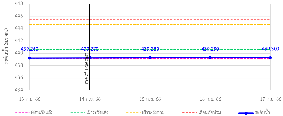
TC030114 สะพานพ่อบุณเมืองรามหาราช ต.แม่ยาว อ.เมืองเชียงราย จ.เชียงราย
