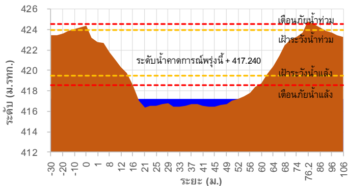
TC 030318 สะพานบ้านป่ารก
