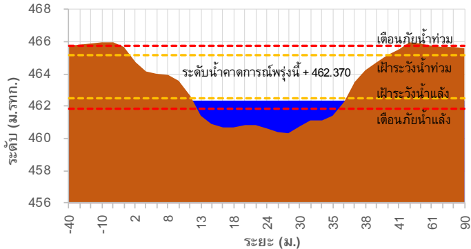
TC 030114 สะพานพอขุนเมืองรามหาราช
