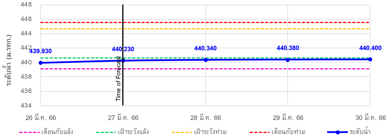
TC 030114 สะพานพ่อนเมืองรายมหาราช ต.แม่ยาว อ.เมืองเชียงราย จ.เชียงราย
