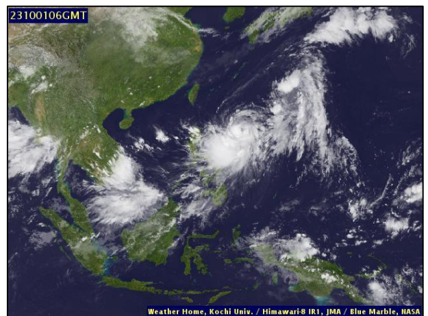
ภาพถ่ายดาวเทียม วันที่ ๑ ต.ค. ๖๖ เวลา ๑๓.๐๐ น.
