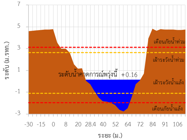
TC191911 สะพานวัดท่าแพ
