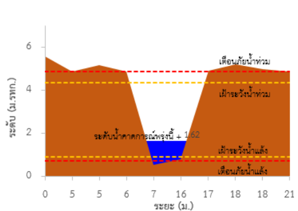
TC220605 สะพานตำราง
