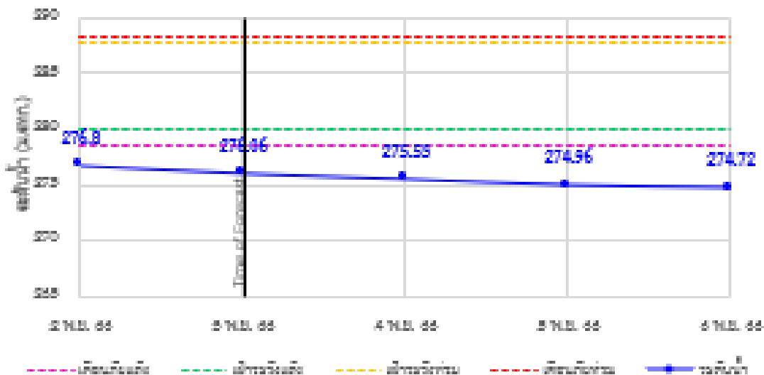
TC011703 สะพานข้ามน้ำแม่ยวม อ.พอรัง อ.แม่ฮ่องสอน จ.ตาก
