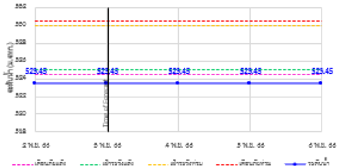
TC010806 สะพานบ้านชนช้าง อ.ชนช้าง จ.ขอนแก่น
