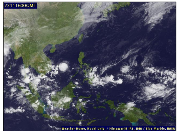
ภาพถ่ายดาวเทียม วันที่ ๑๖ พ.ย. ๖๖ เวลา ๐๗.๐๐ น.
