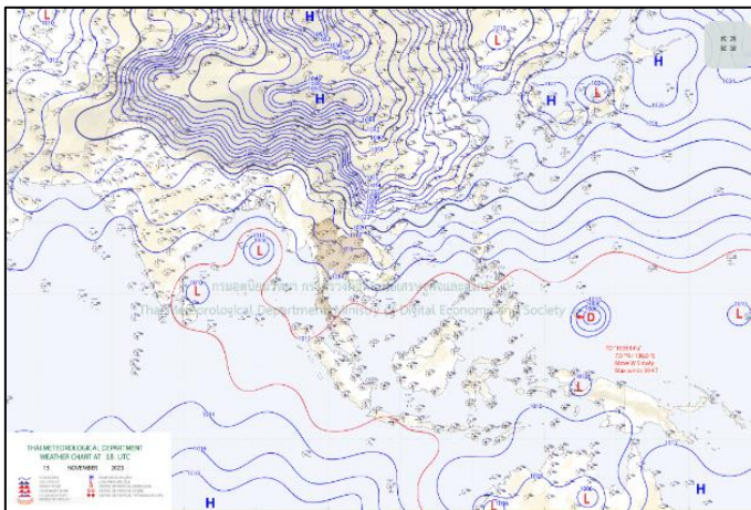
แผนที่อากาศ วันที่ ๑๖ พ.ย. ๒๕๖๖ เวลา ๐๑.๐๐ น.
