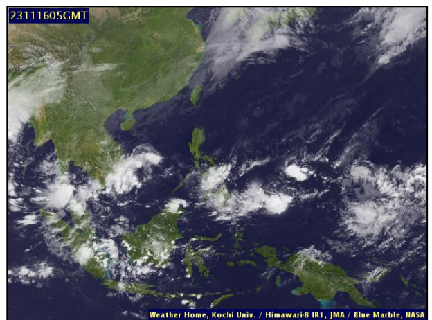
ภาพถ่ายดาวเทียม วันที่ ๑๖ พ.ย. ๖๖ เวลา ๑๒.๐๐ น.
