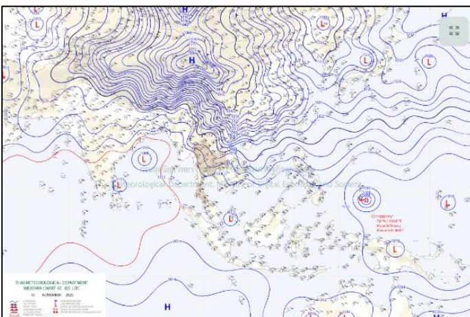
แผนที่อากาศ วันที่ ๑๖ พ.ย. ๒๕๖๖ เวลา ๐๗.๐๐ น.
