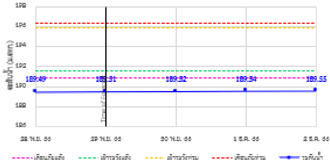
TC010605 สถานีบ้านป่าอ้อ อ.มาบป๋วย จ.แม่ฮ่องสอน
