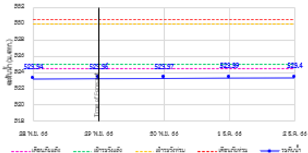
TC010806 สะพานบ้านชนขาม อ.ชนขาม จ.แม่ฮ่องสอน
