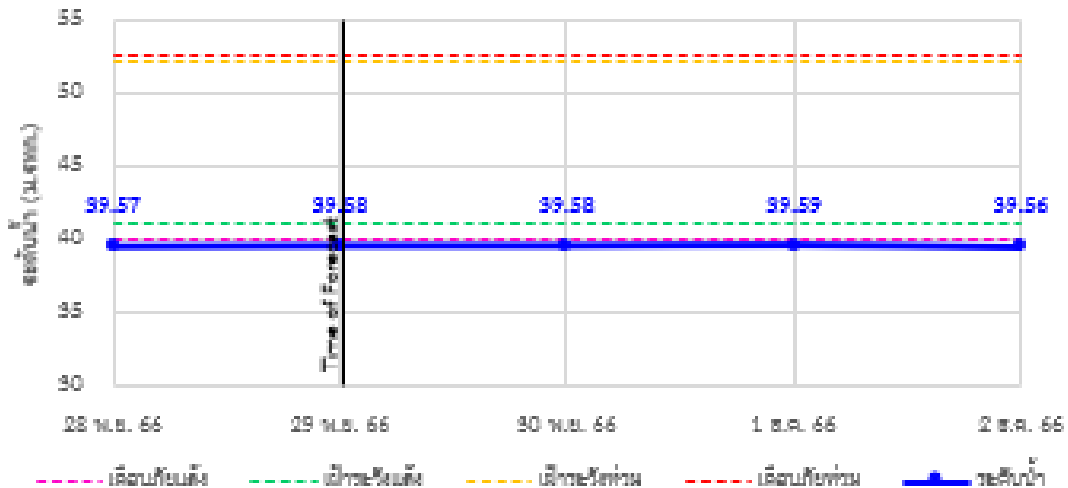
TC140605 สะพาน กฟผ.เจทีศ อ.ช่องสะแก อ.เมือง จ.กาญจนบุรี
