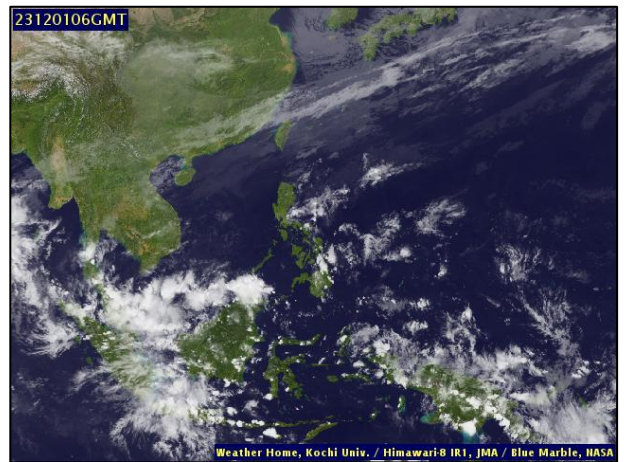
ภาพถ่ายดาวเทียม วันที่ ๑ ธ.ค. ๖๖ เวลา ๑๓.๐๐ น.
