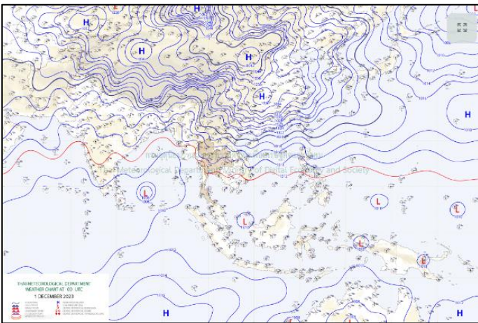
แผนที่อากาศ วันที่ ๑ ธ.ค. ๒๕๖๖ เวลา ๐๗.๐๐ น.
