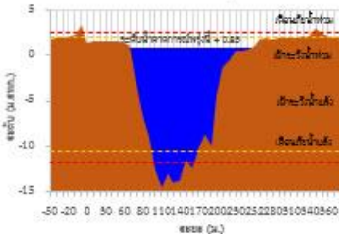
TC140104 สะพานสมเด็จพระศรีสุทธานนท์
