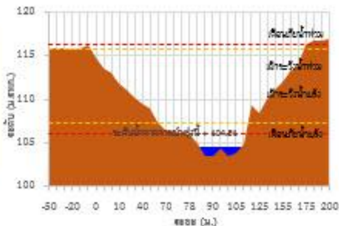
TC141101 สะพานคณาจารย์
