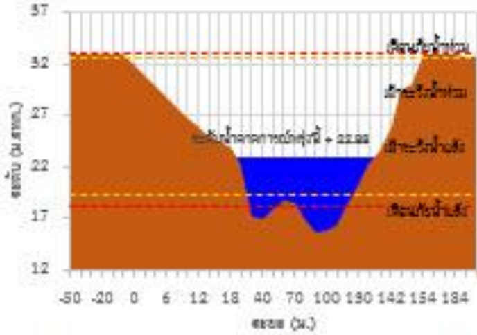
TC140102 สะพานเฉลิมพระเกียรติ 60 พรรช นามหาชวินี
