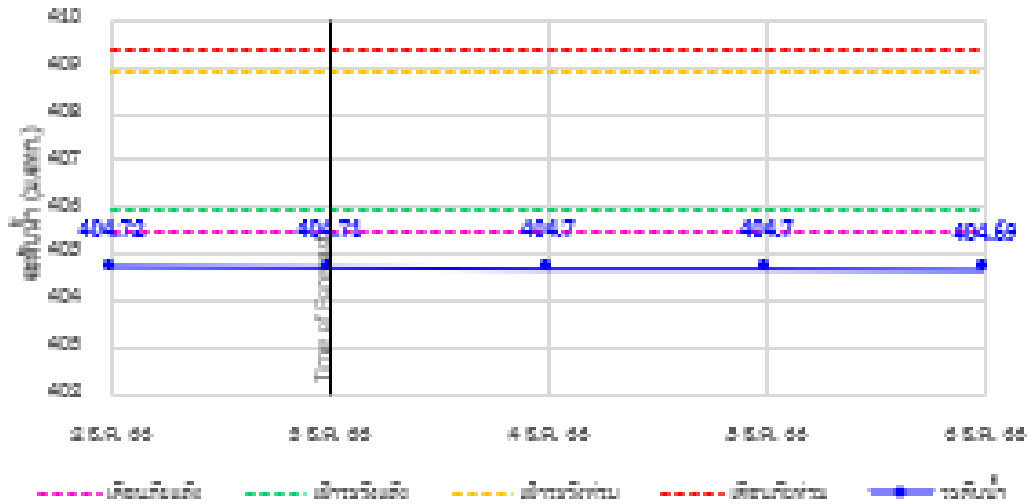
TC010703 สะพานบ้านแม่หิน อ.ชนบท จ.แม่ฮ่องสอน
