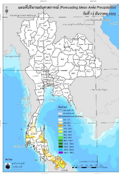
ปริมาณฝนคาดการณ์ในวันที่ 13 ธันวาคม 2566
