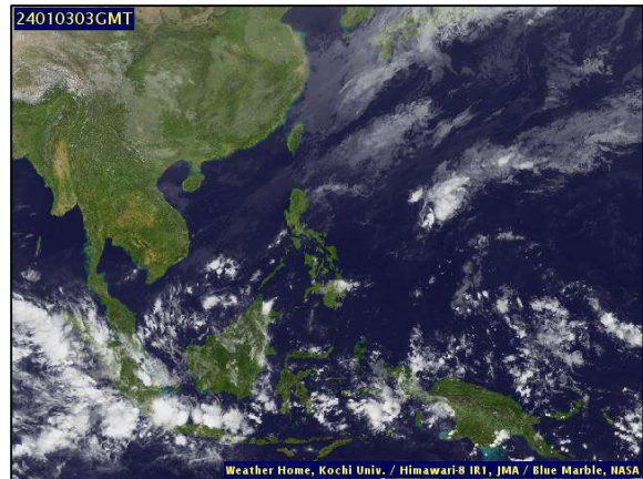
ภาพถ่ายดาวเทียม วันที่ ๓ ม.ค. ๖๗ เวลา ๑๐.๐๐ น.
