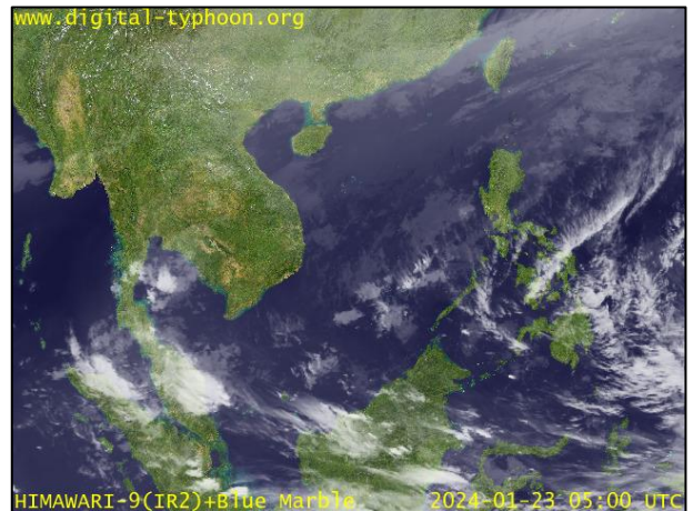
ภาพถ่ายดาวเทียม วันที่ ๒๓ ม.ค. ๒๕๖๗ เวลา ๑๒.๐๐ น.
