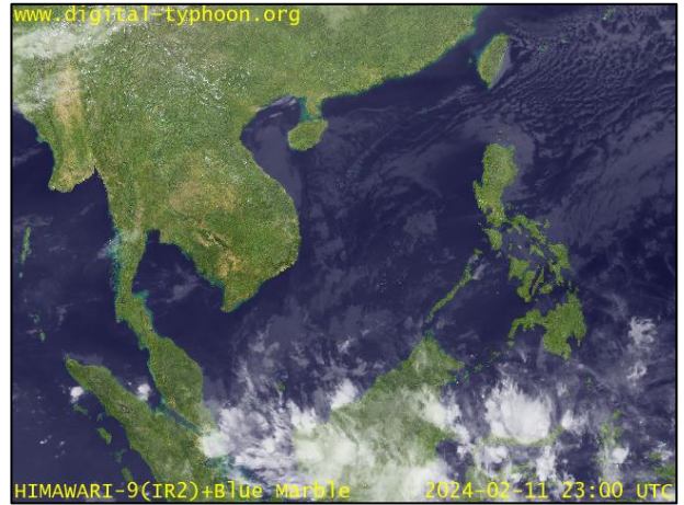
ภาพถ่ายดาวเทียม วันที่ ๑๒ ก.พ. ๒๕๖๗ เวลา ๐๖.๐๐ น.
