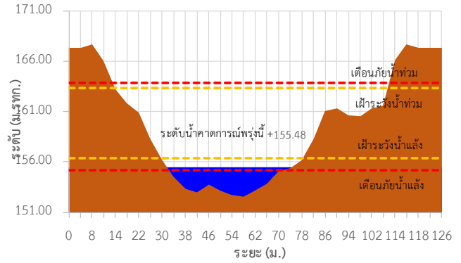
TC031902 สะพานคอนเซียงยืน ต.ดงเย็น อ.บ้านดุง จ.อุดรธานี
