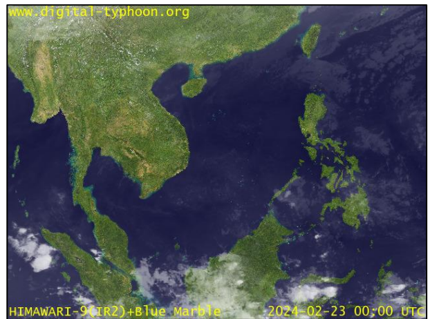
ภาพถ่ายดาวเทียม วันที่ ๒๓ ก.พ. ๒๕๖๗ เวลา ๐๗.๐๐ น.
