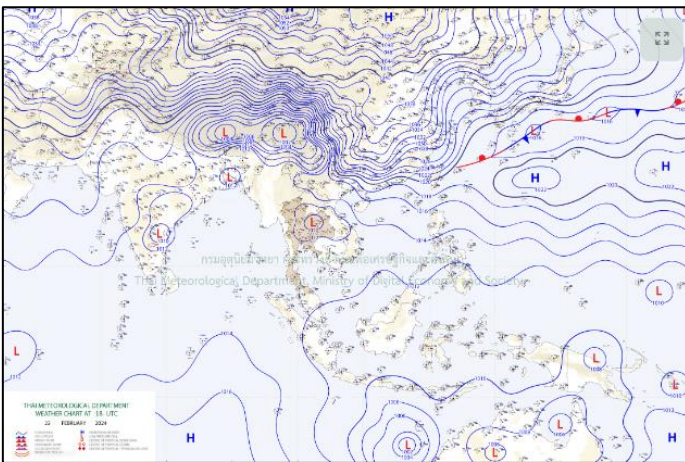
แผนที่อากาศ วันที่ ๒๓ ก.พ. ๒๕๖๗ เวลา ๐๑.๐๐ น.
