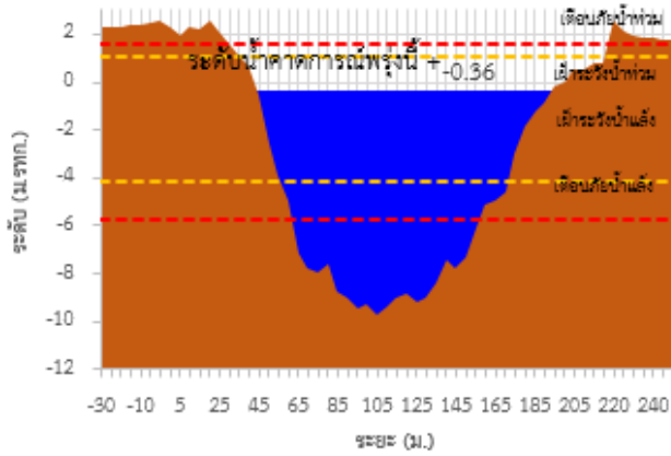
TC191001 สะพานข้ามแม่น้ำตาปี ตลาดจวง
