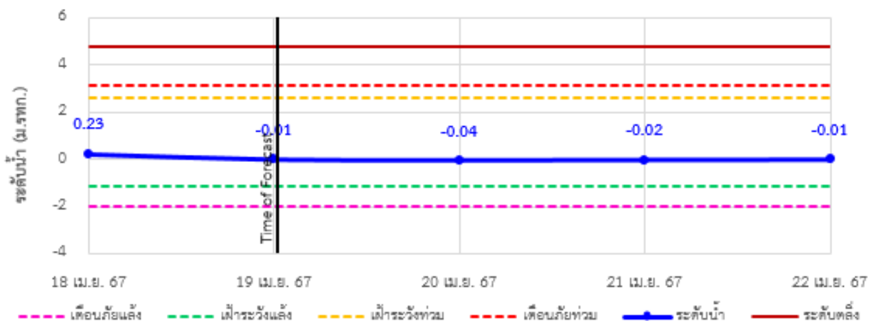
TC191802 สะพานบ้านไร่เหล็ก ค.นบพิศำ อ.นบพิศำ จ.นครศรีธรรมราช
