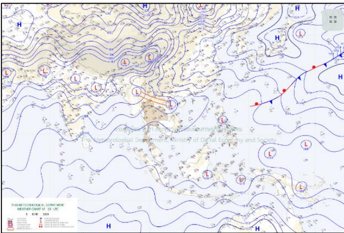
แผนที่อากาศ วันที่ ๖ มิ.ย. ๒๕๖๗ เวลา ๐๑.๐๐ น.
