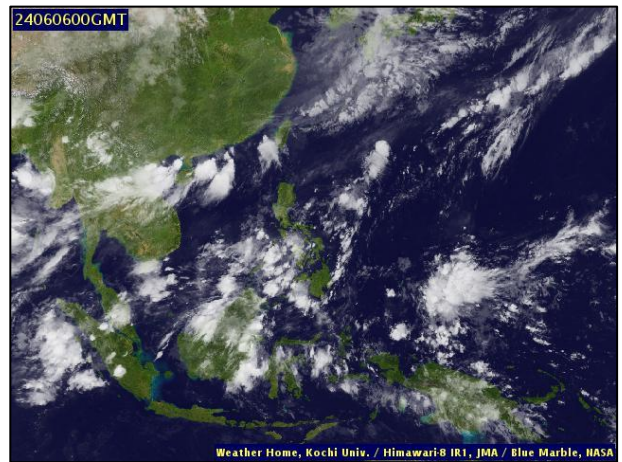
ภาพถ่ายดาวเทียม วันที่ ๖ มิ.ย. ๒๕๖๗ เวลา ๐๗.๐๐ น.
