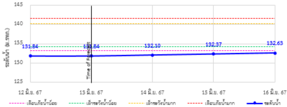
TC032705 สะพาน นพ.4059 ค.ท่าบ่อสงคราม อ.ศรีสงคราม จ.นครพนม
