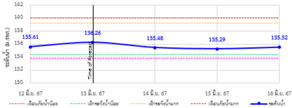
TC032501 สะพานบ้านหนองบัว ค.บ้านข่า อ.ศรีสงคราม จ.นครพนม
