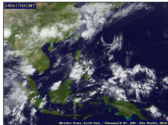
ภาพถ่ายดาวเทียม วันที่ ๑๗ มิ.ย. ๒๕๖๗ เวลา ๐๗.๐๐ น.
