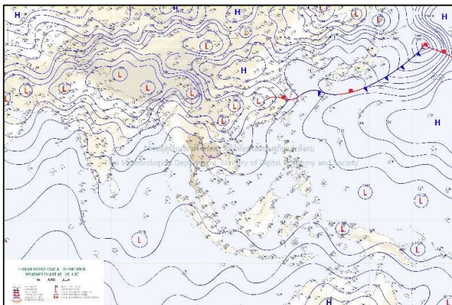
แผนที่อากาศ วันที่ ๑๗ มิ.ย. ๒๕๖๗ เวลา ๐๑.๐๐ น.
