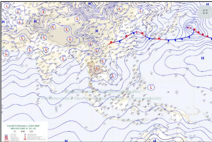
แผนที่อากาศ วันที่ ๒๒ มิ.ย. ๒๕๖๗ เวลา ๐๗.๐๐ น.
