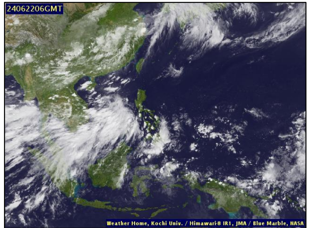
ภาพถ่ายดาวเทียม วันที่ ๒๒ มิ.ย. ๒๕๖๗ เวลา ๑๓.๐๐ น.
