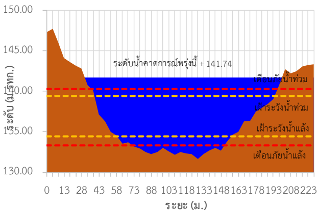
TC032705 สะพาน นพ.4059 ต.ท่าบ่อสงคราม อ.ศรีสงคราม จ.นคร
