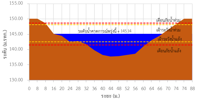
TC032501 สะพานบ้านหนองบัว ต.บ้านข่า อ.ศรีสงคราม จ.นครพนม
