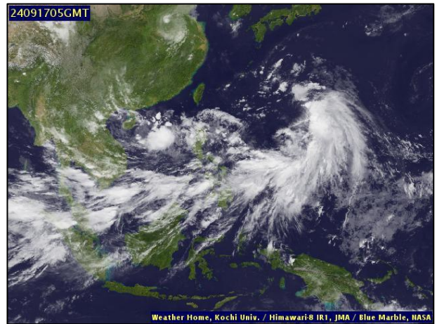
ภาพถ่ายดาวเทียม วันที่ ๑๗ ก.ย. ๒๕๖๗ เวลา ๑๒.๐๐ น.
