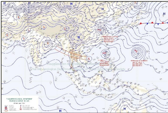
แผนที่อากาศ วันที่ ๑๗ ก.ย. ๒๕๖๗ เวลา ๐๗.๐๐ น.
