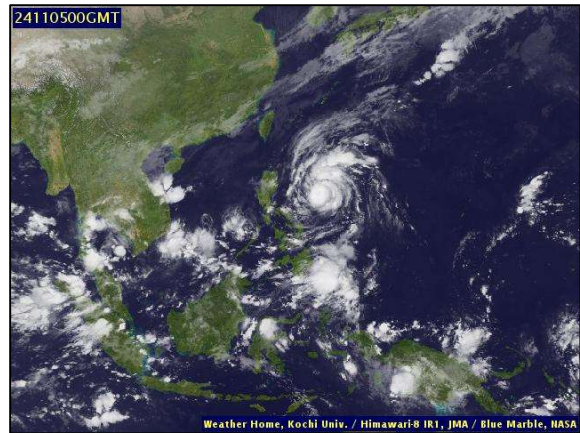
ภาพถ่ายดาวเทียม วันที่ ๕ พ.ย. ๒๕๖๗ เวลา ๐๗.๐๐ น.
