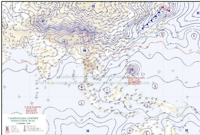
แผนที่อากาศ วันที่ ๑๗ พ.ย. ๒๕๖๗ เวลา ๐๑.๐๐ น.
