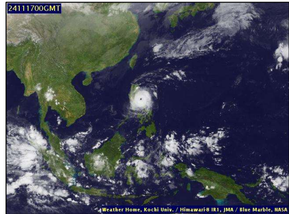
ภาพถ่ายดาวเทียม วันที่ ๑๗ พ.ย. ๒๕๖๗ เวลา ๐๗.๐๐ น.
