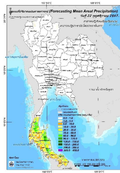
ปริมาณฝนคาดการณ์ในวันที่ 21 พฤศจิกายน 2567 ปริมาณฝนคาดการณ์ในวันที่ 22 พฤศจิกายน 2567
