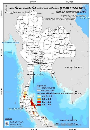
วันที่ 22 พ.ย. 2567 (03:00 น.) วันที่ 22 พ.ย. 2567 (15:00 น.) วันที่ 23 พ.ย. 2567 (03:00 น.)
