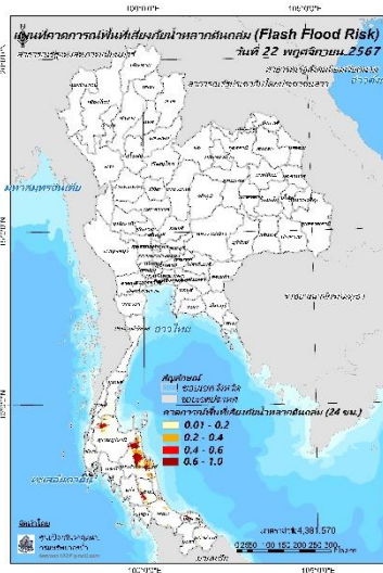
วันที่ 22 พ.ย. 2567 (03:00 น.) วันที่ 22 พ.ย. 2567 (15:00 น.) วันที่ 23 พ.ย. 2567 (03:00 น.)
