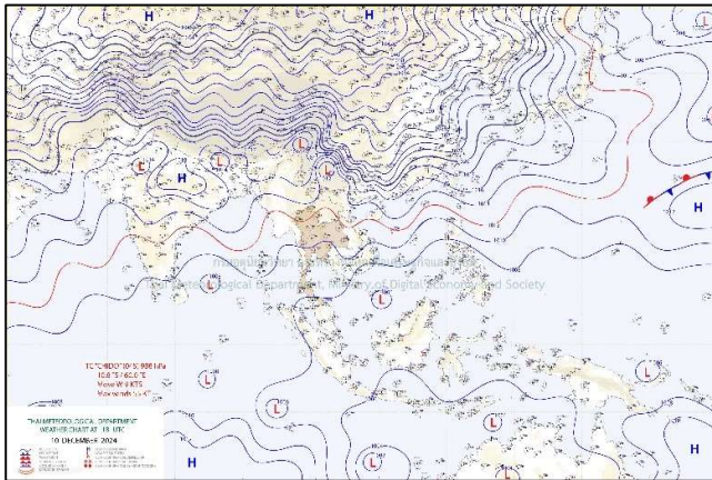
แผนที่อากาศ วันที่ ๑๑ ธ.ค. ๒๕๖๗ เวลา ๐๑.๐๐ น.
