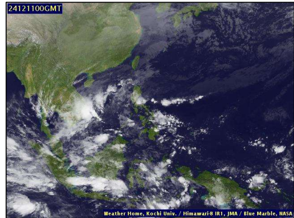
ภาพถ่ายดาวเทียม วันที่ ๑๑ ธ.ค. ๒๕๖๗ เวลา ๐๗.๐๐ น.
