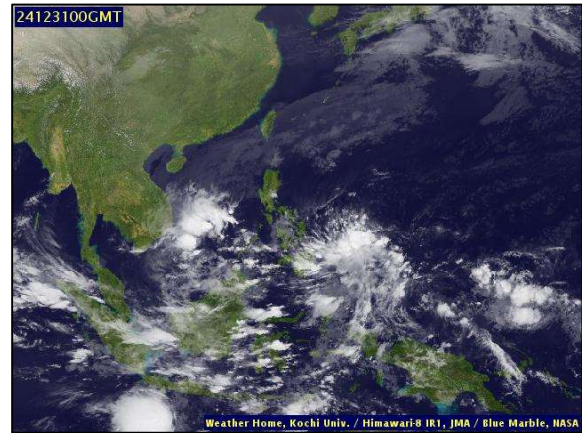
ภาพถ่ายดาวเทียม วันที่ ๓๑ ธ.ค. ๒๕๖๗ เวลา ๐๗.๐๐ น.
