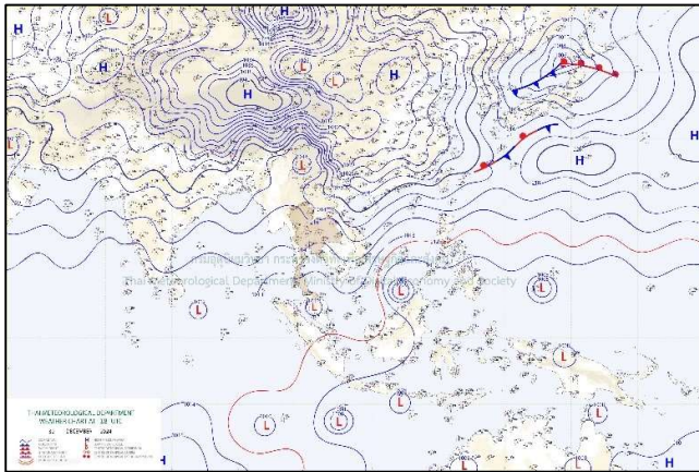
แผนที่อากาศ วันที่ ๓๑ ธ.ค. ๒๕๖๗ เวลา ๐๑.๐๐ น.
