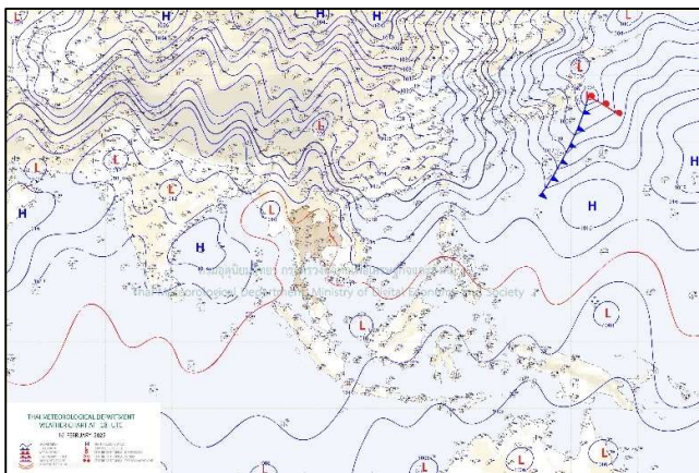
แผนที่อากาศ วันที่ ๑๗ ก.พ. ๒๕๖๘ เวลา ๐๑.๐๐ น.
