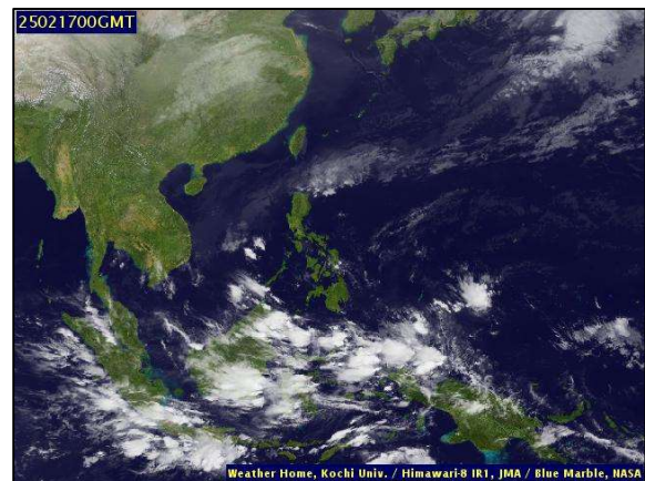
ภาพถ่ายดาวเทียม วันที่ ๑๗ ก.พ. ๒๕๖๘ เวลา ๐๗.๐๐ น.
