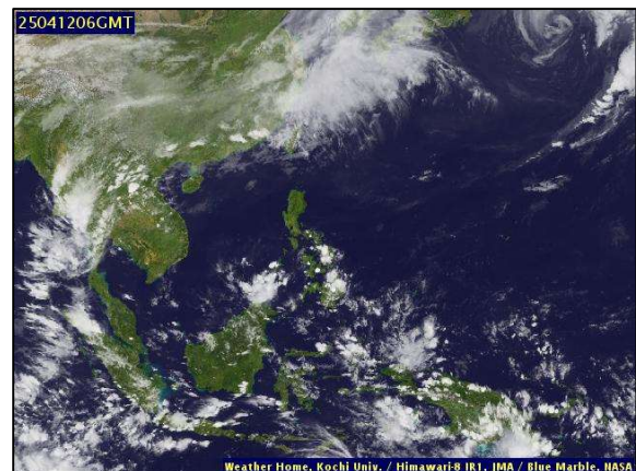
ภาพถ่ายดาวเทียม วันที่ ๑๒ เม.ย. ๒๕๖๘ เวลา ๑๓.๐๐ น.
