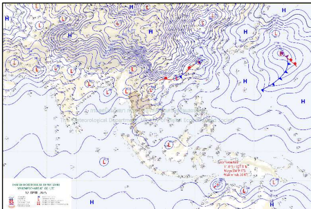
แผนที่อากาศ วันที่ ๑๒ เม.ย. ๒๕๖๘ เวลา ๐๗.๐๐ น.
